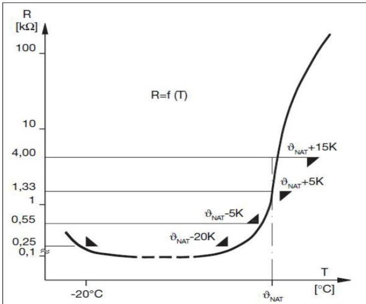
Rys. 1 – Charakterystyka czujnika PTC.
