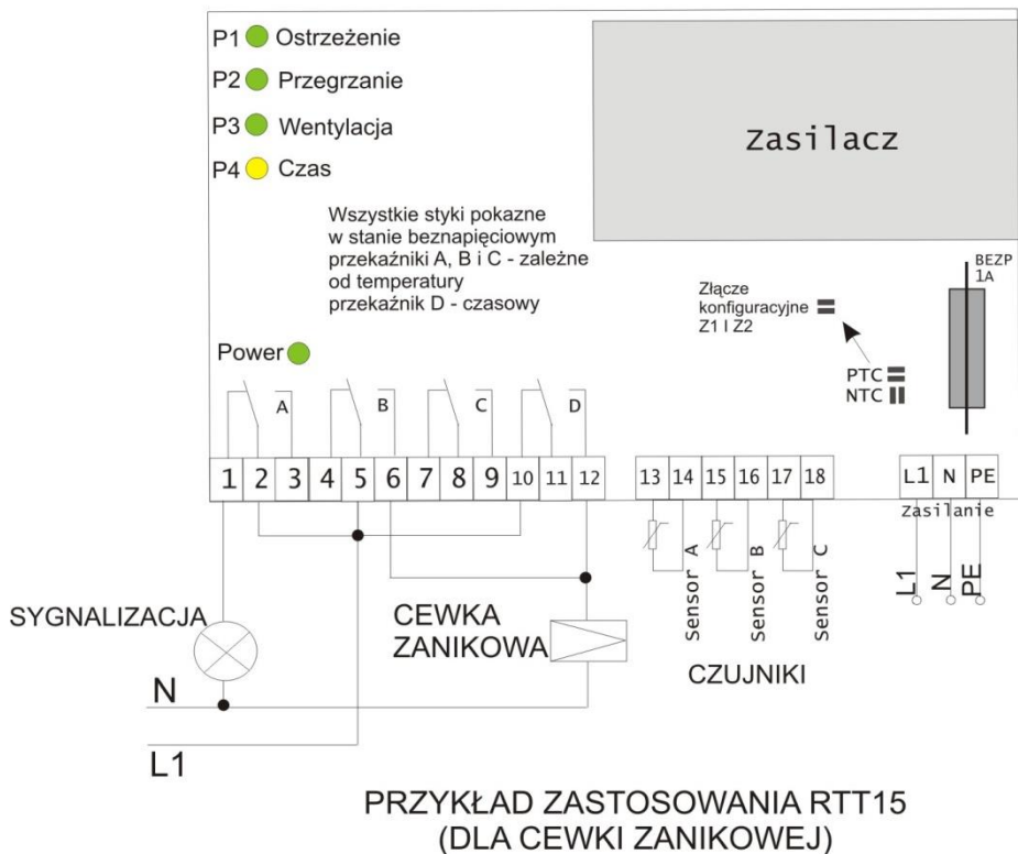
Rys. 3 – Przykłady zastosowania układu RTT-15 wyposażonego w 2 czujniki temperatury PTC z wyłącznikiem wyposażonym w cewkę zanikową lub wybijakową.
