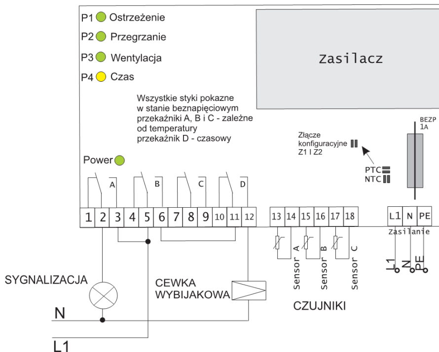
Rys. 4 – Przykłady zastosowania układu RTT-15 wyposażonego w 2 czujniki temperatury PTC z wyłącznikiem wyposażonym w cewkę wybijkową.
