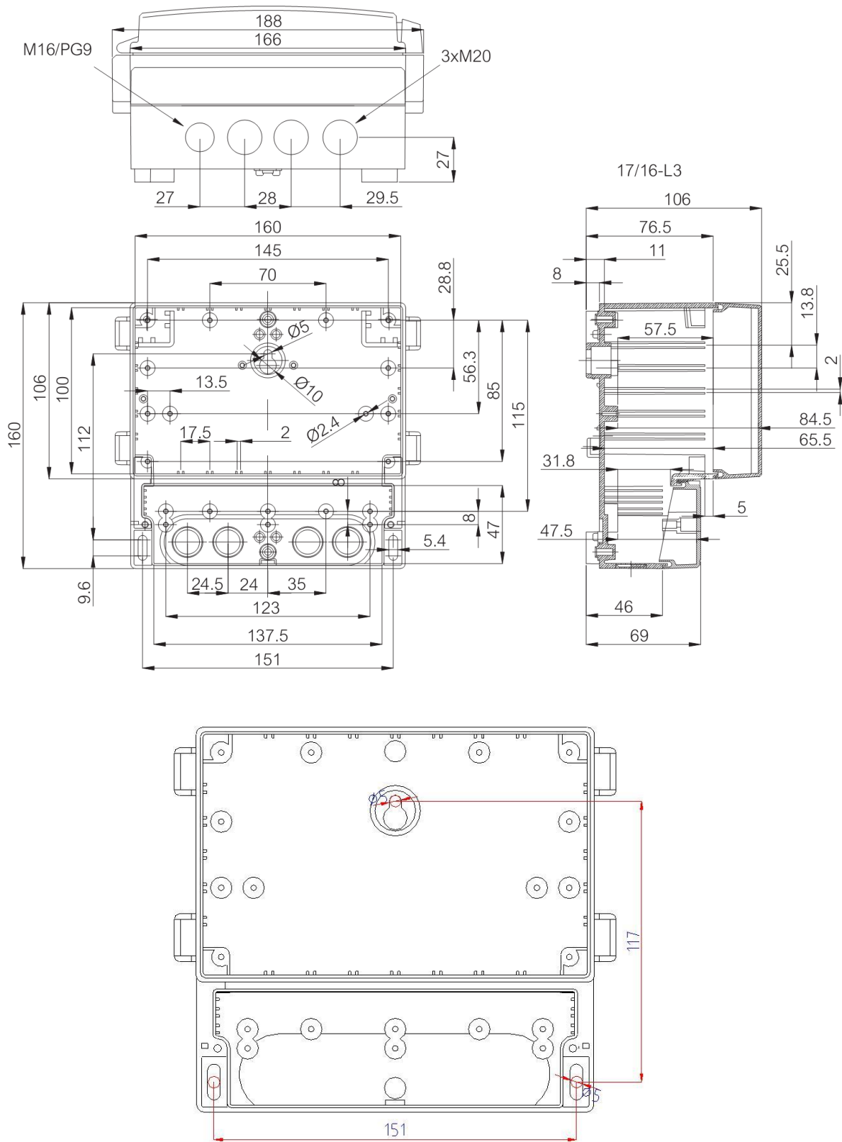
Rys. 2 - Wymiary obudowy oraz rozstaw otworów mocujących
