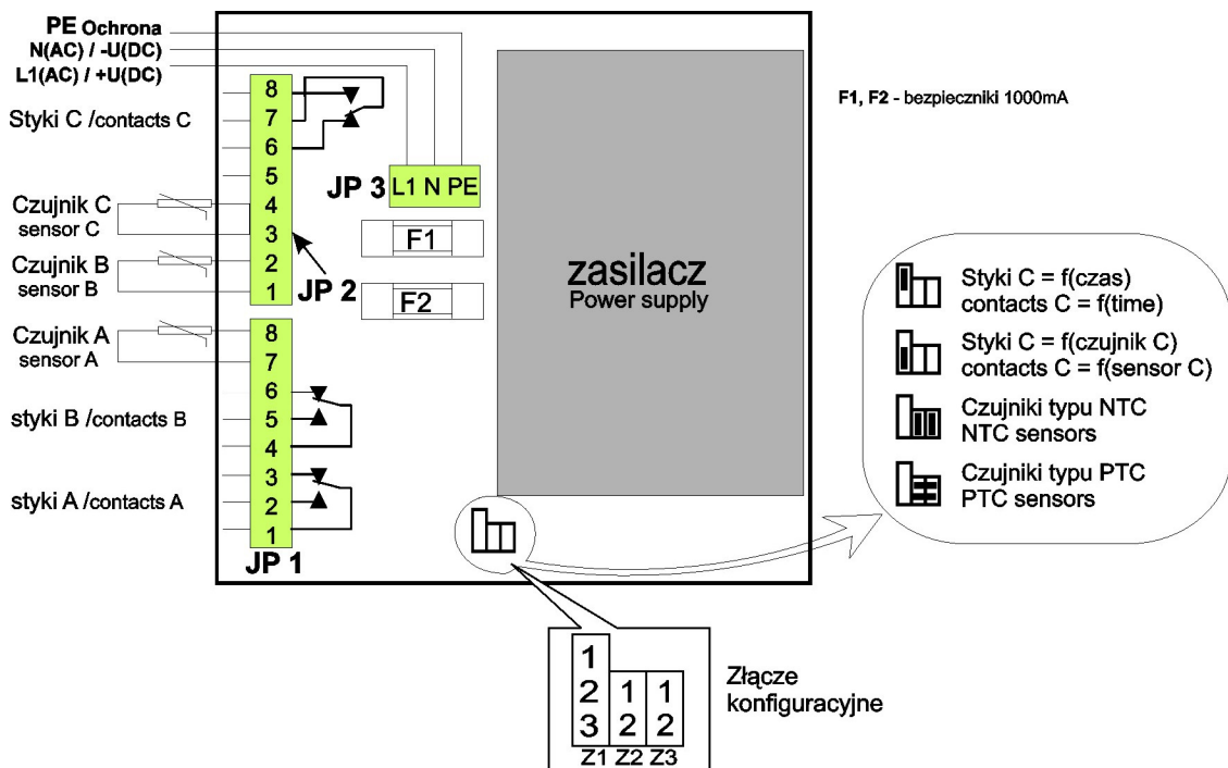
Rys. 2 – schemat podłączenia RTT-4/2 i opis złączy konfiguracyjnych
