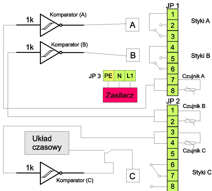
Rys. 1 – schemat blokowy układu RTT 4/2
