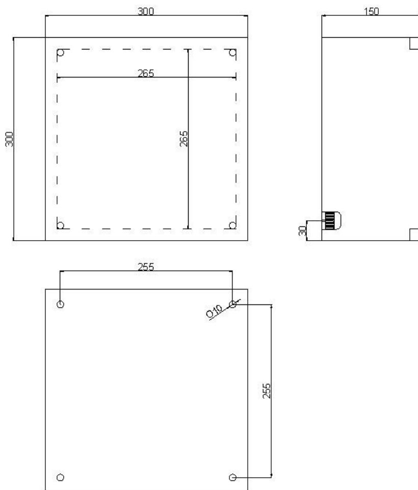
Rys. 5 – Wymiary obudowy RTT-4/2.
